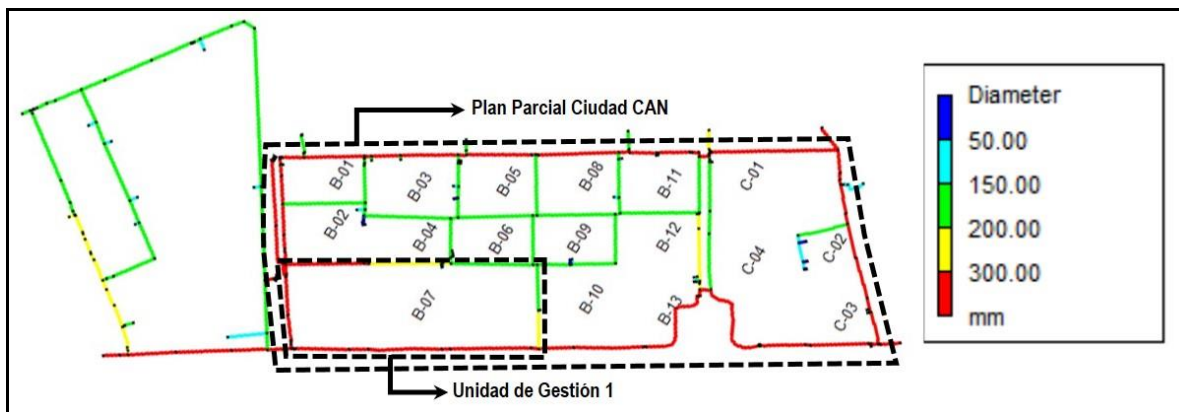
Ilustración No. 4 – Diámetros tubería acueducto en diseño conceptual del P.P. Ciudad CAN. Fuente: Elaboración propia, ANIM 2020.
