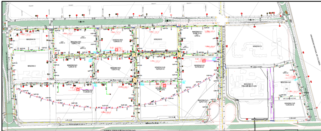
Ilustración No. 6 – Red de alumbrado público conceptual para el P.P. Ciudad CAN.
